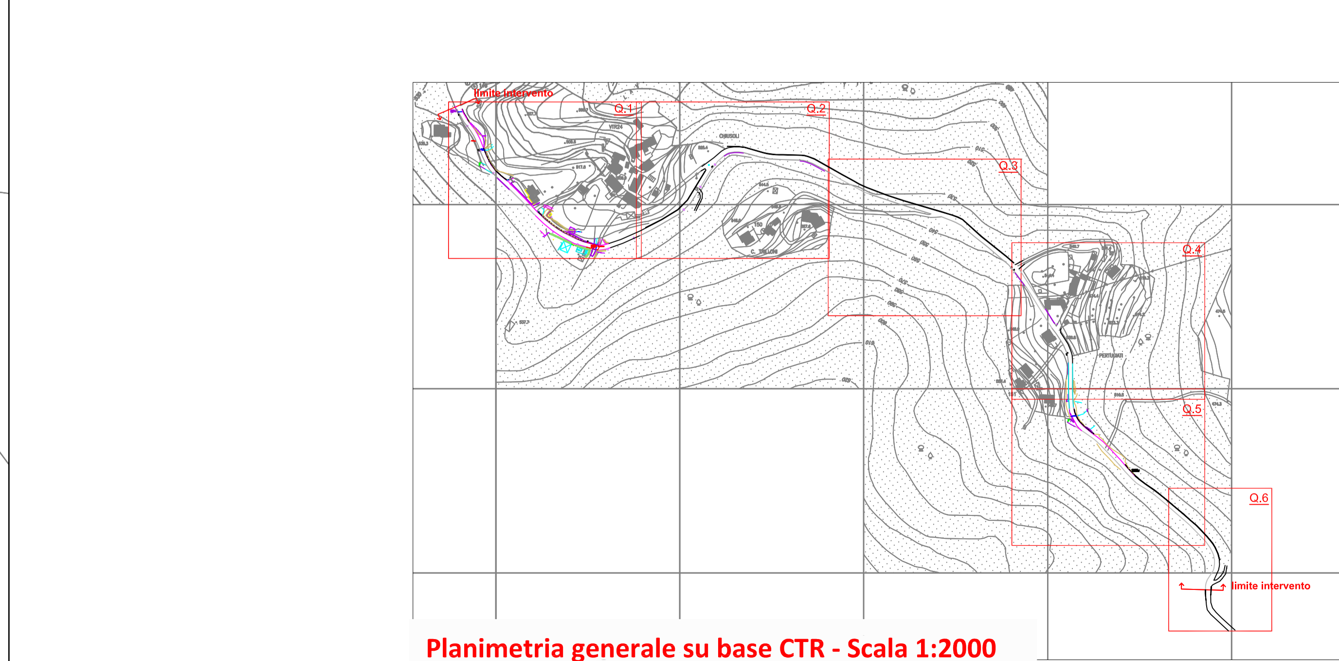
Planimetria generale su base CTR - Scala 1:2000
