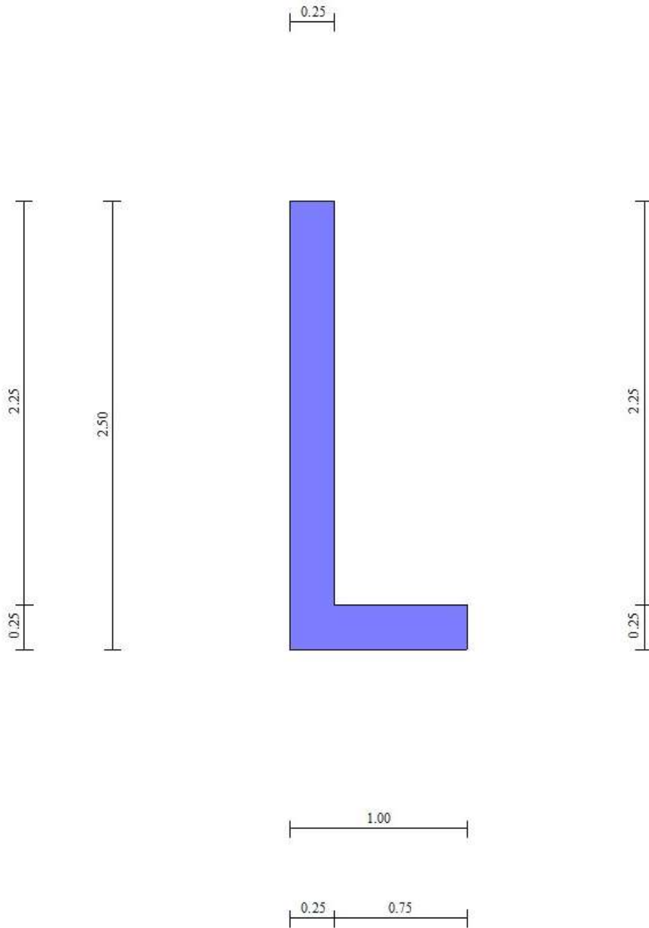
Fig. 3 - Sezione quotata del muro
