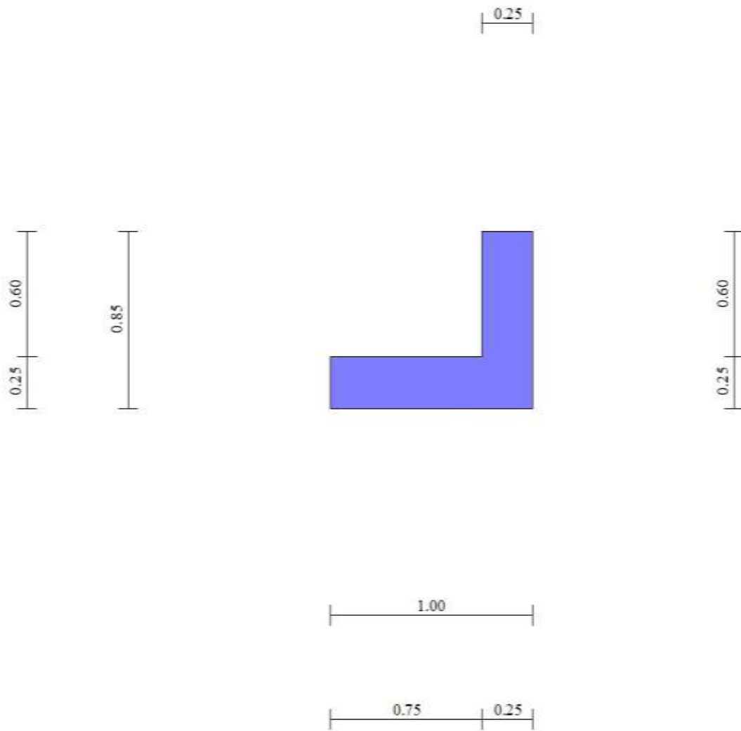
Fig. 5 - Sezione quotata del muro
